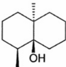
Geosmin
